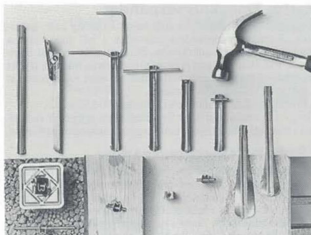
Klemit lättbetonginfästning, typer
