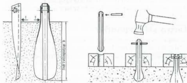
Klemits expansion efter islagning
